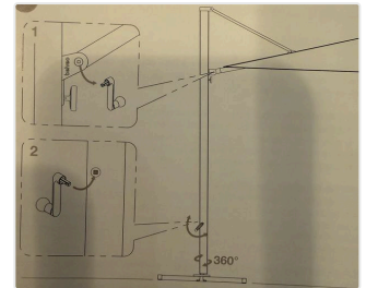
Pour le faire pivoter sur 360° – débloquez le levier au pied, tournez, puis rebloquez.
